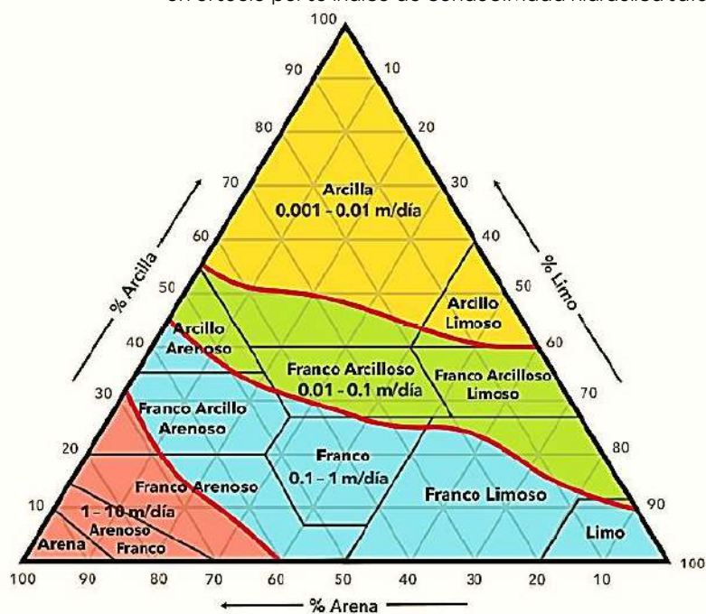
Ilustración 36. Evaluación de la capacidad de infiltración de Agua en el suelo por su índice de conductividad hidráulica saturada (m/día)
