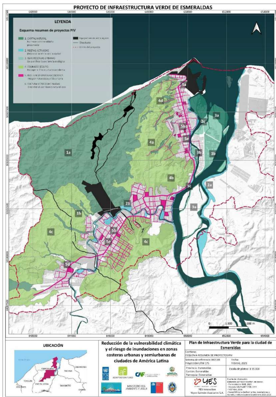
Ilustración 93. Propuesta de Infraestructura Verde
